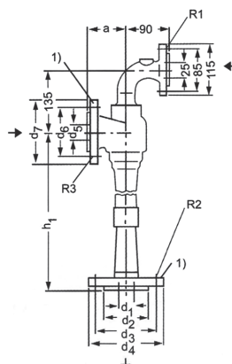
大气喷射器 Gas ejector 2BP5
