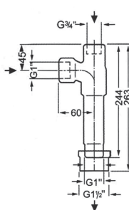
大气喷射器 Gas ejector 2BP1 07.
